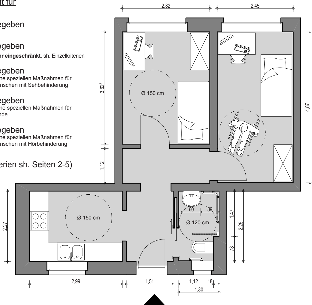
2er-WG Zimmer 00.03 / 00.04
